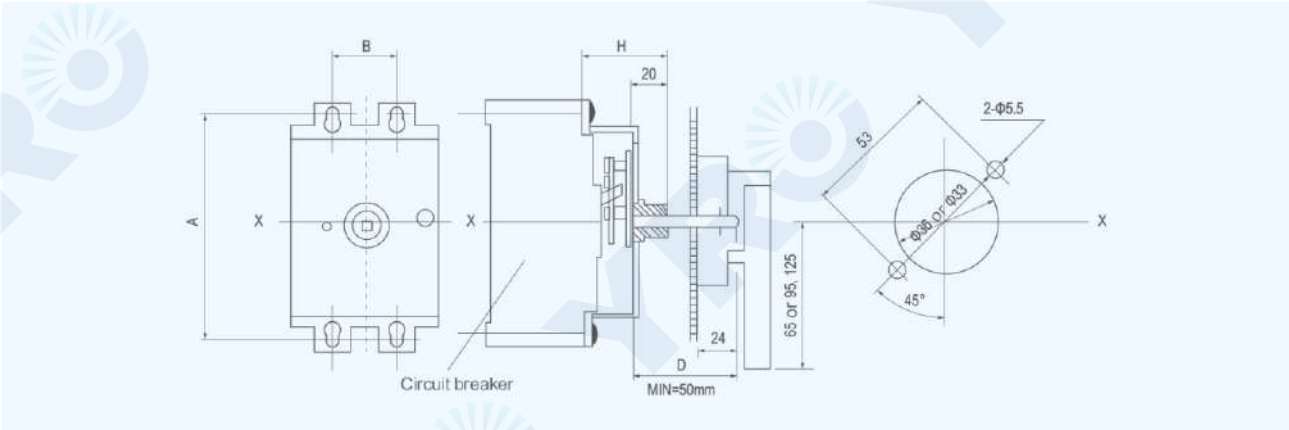
Schematic of CS1-A handle
